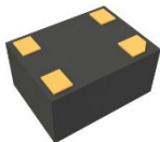
2.4 GHz 芯片天线 ACAG0201-2450-T 尺寸 2.0 x 1.25mm 厚度 0.6mm
