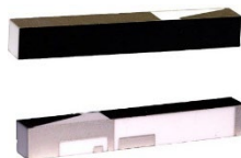
SAW 滤波器蜂窝通信 ADSTS5A2-1CHM011M 尺寸1.1 x 0.9mm 厚度 0.5mm
