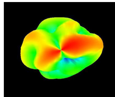
2170 MHz
